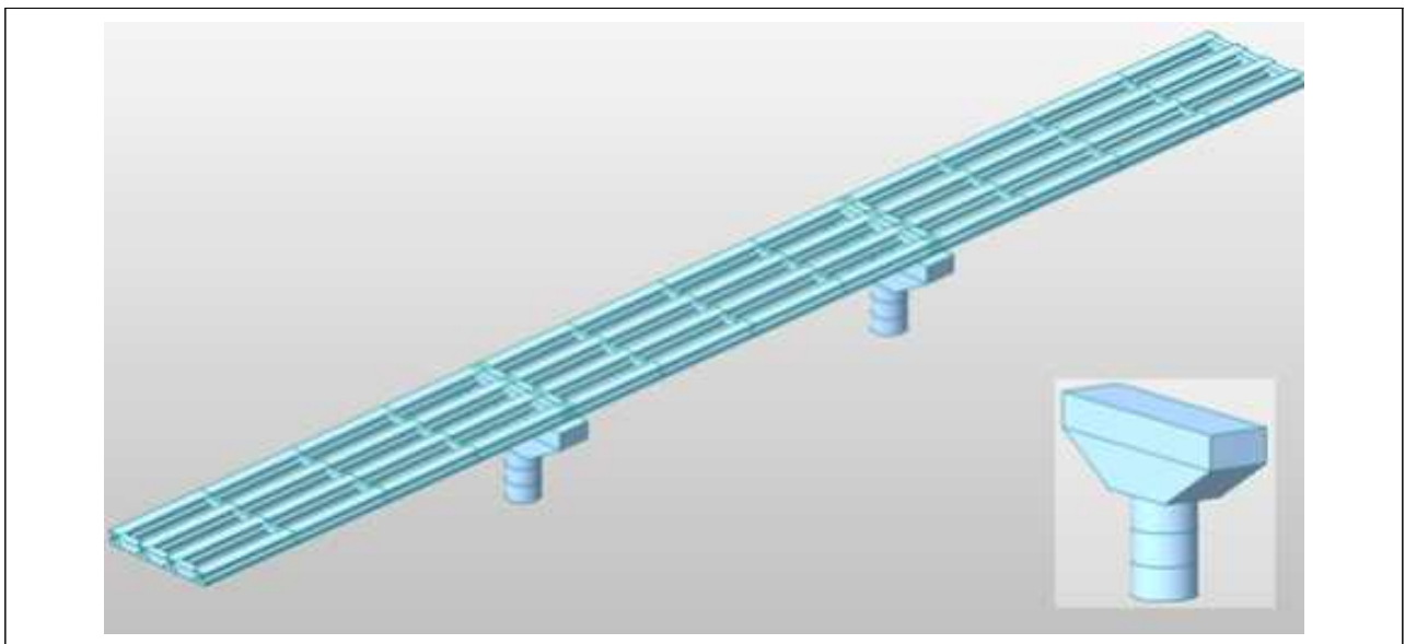
【그림 4.17】 수기2교(하) 교량 구조해석 모델링
