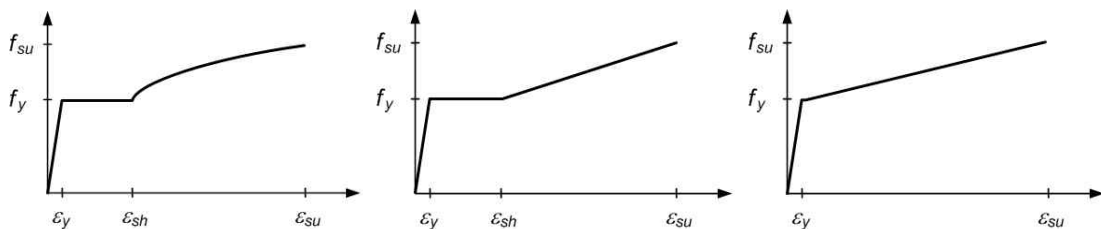
【그림 4.3】 철근의 강도 및 변형률
