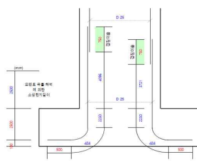
소성인지부 겹이음 검토
