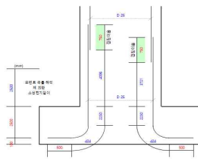
소성힌지부 겹이음 검토
