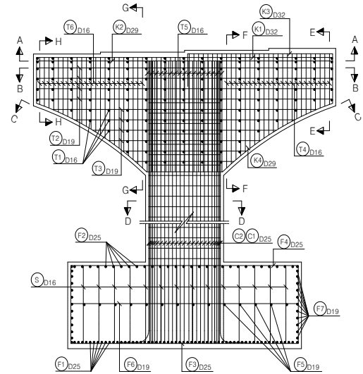
【그림 4.16】 수기2교(하) 철근 상세도
