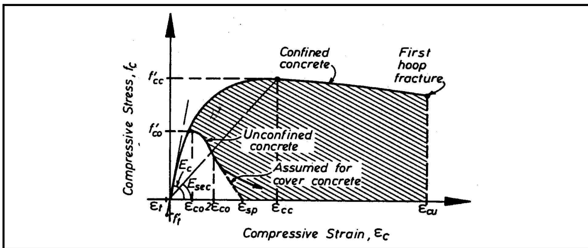
【그림 4.2】 Mander 등의 콘크리트 압축응력 변형률 모델
