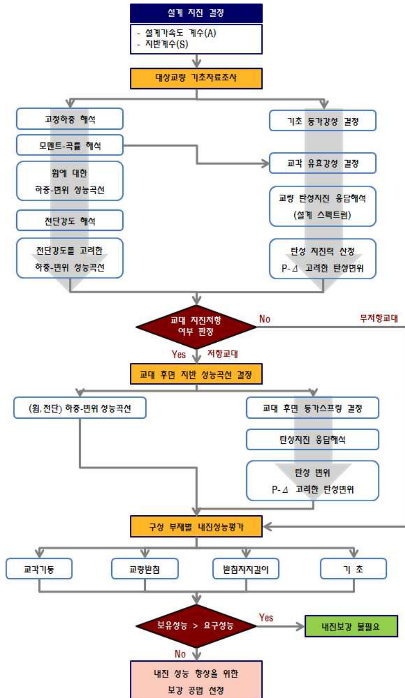
【그림 4.1】 내진성능평가 흐름도
