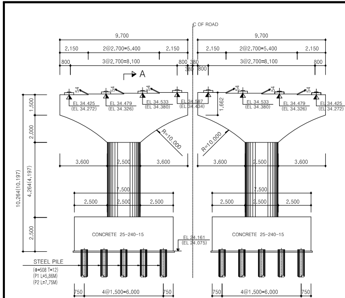
【그림 4.15】 수기2교(하) 교각 일반도
